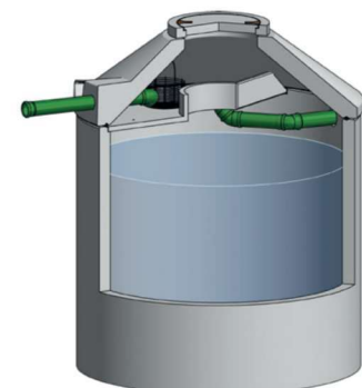
Zulaufhöhe 570 mm, Ablaufhöhe 910 mm unterhalb der Schachtabdeckung bis Rohrsohle.
