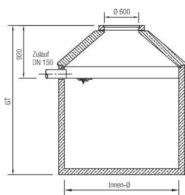
Abwassersammelgrube
