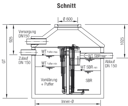
Technische Daten SanoClean S classicline als Kompletanlage in Beton
