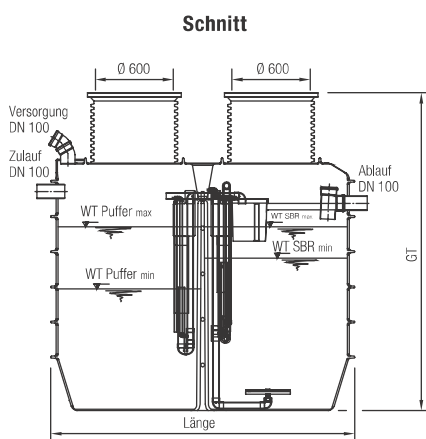
Technische Daten SanoClean S classicline als Kompletanlage in PE
